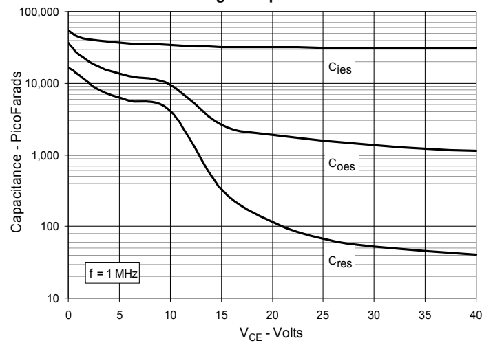
Fig. 8. Capacitance
