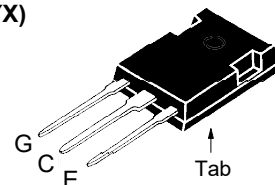
TO-247PLUS-HV (IXYX..HV)
