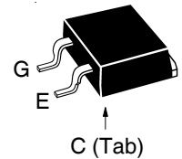
TO-263HV (IXYA..HV)
