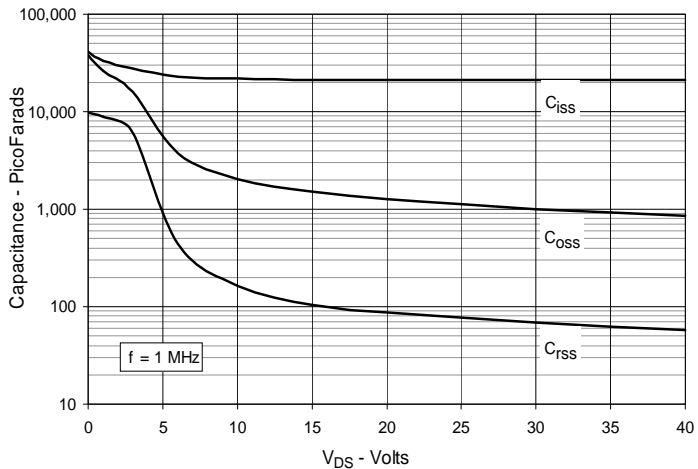
Fig. 11. Capacitance
