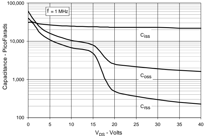
Fig. 11. Capacitance
