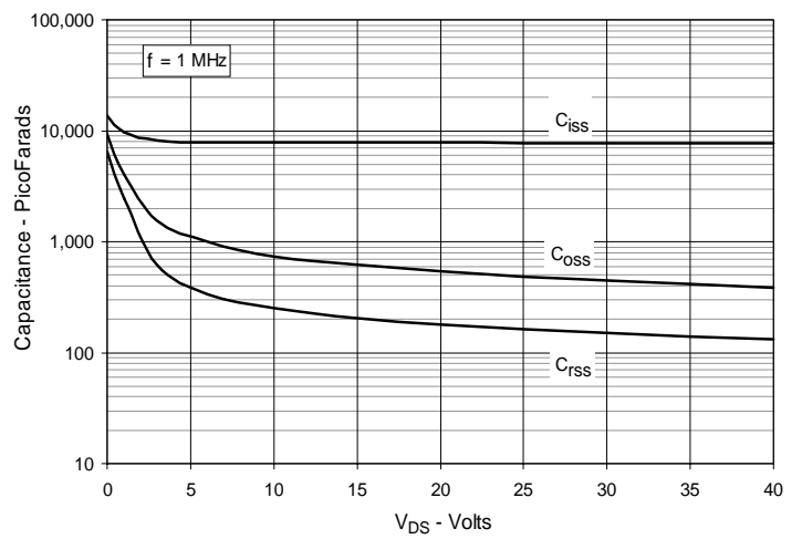
Fig. 10. Capacitance
