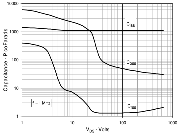
Fig. 12. Capacitance
