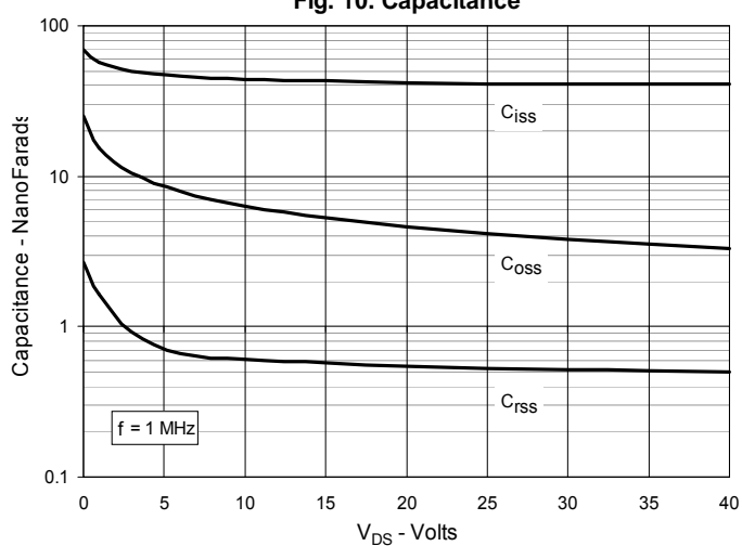
Fig. 10. Capacitance
