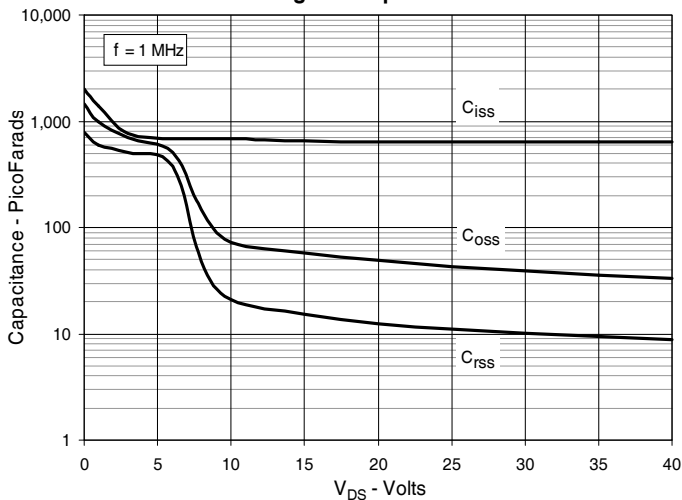
Fig. 13. Capacitance
